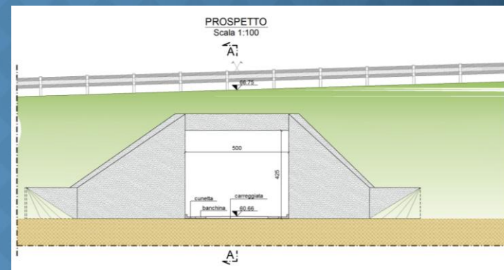
Sezione Sovrappasso
