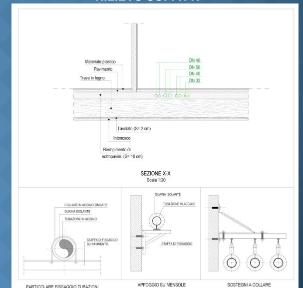
SEZIONE SOTTOTETTO – Impianti di riscaldamento e condizionamento
